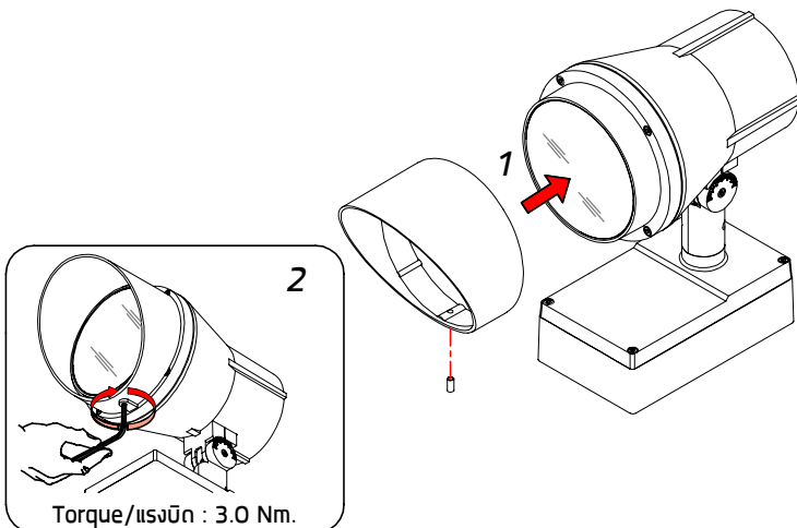
Part-A/ชิ้น-A
