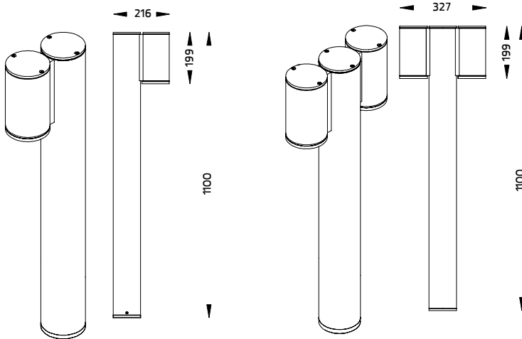
Mini TUBE - Bollard / Single Sided
