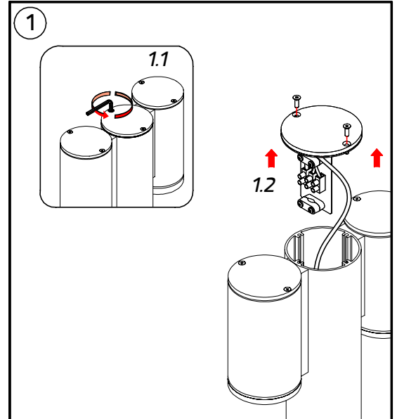
Mini TUBE - Bollard / Double Sided
