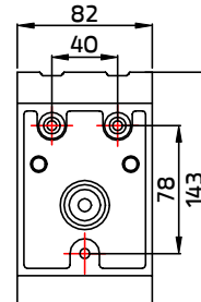
Wall bracket แป้นยึดผนัง OD-5006
