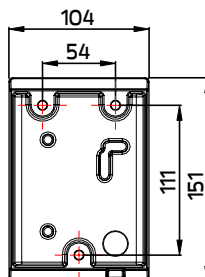
Wall bracket แป้นยึดผนัง OD-5005
