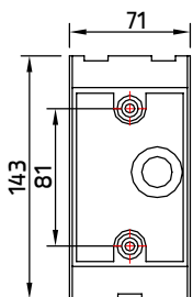
Wall bracket แบบยึดผนัง OD-5001
