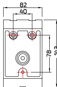
Wall bracket แบบยึดผนัง OD-5003
