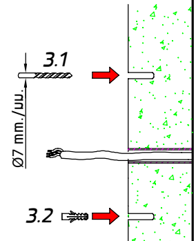
Cable size : 3X1.00 mm. Ø8-13 mm. ขนาดสายไฟ
