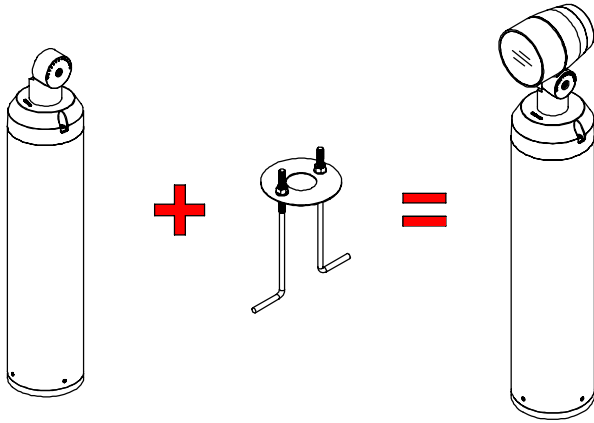
Short Pole. [On/Off] Ordering Code/รหัสสั่งซื้อ : AUN-POL-0188-XX
