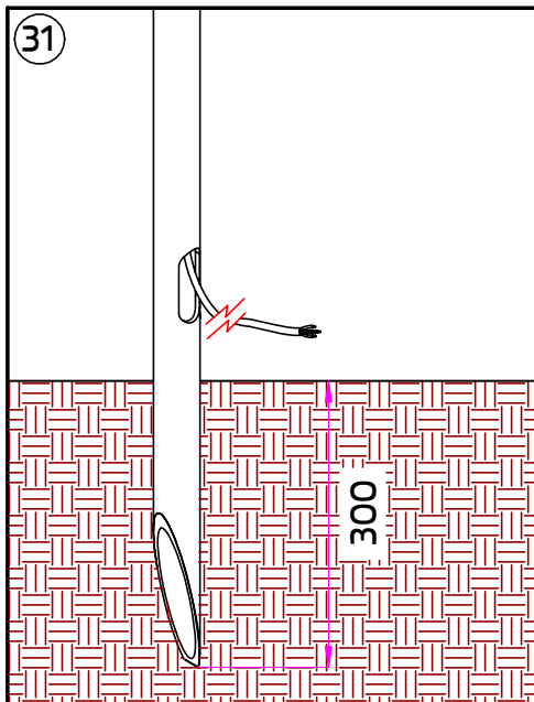
Aluminium Earth Spike L 900mm. [On/Off] Ordering Code/รหัสสั่งซื้อ : AUN-ESP-0021-XX
