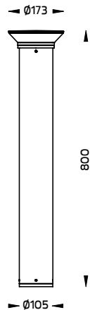
Mini AGAR Prismatic-Bollard / Mini AGAR Opal - Bollard
