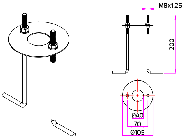
Mini AGAR Prismatic-Bollard / Mini AGAR Opal - Bollard
